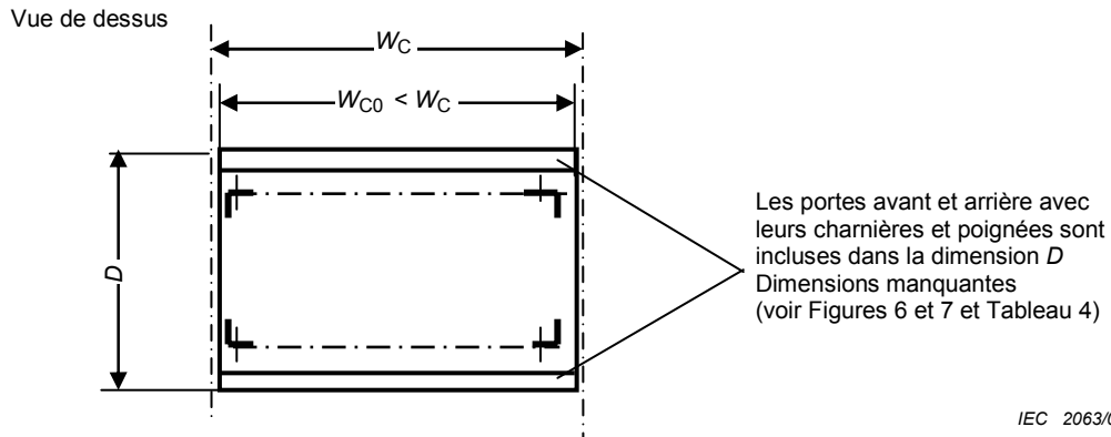
Figure 8 – Dimensions des baies de type B
