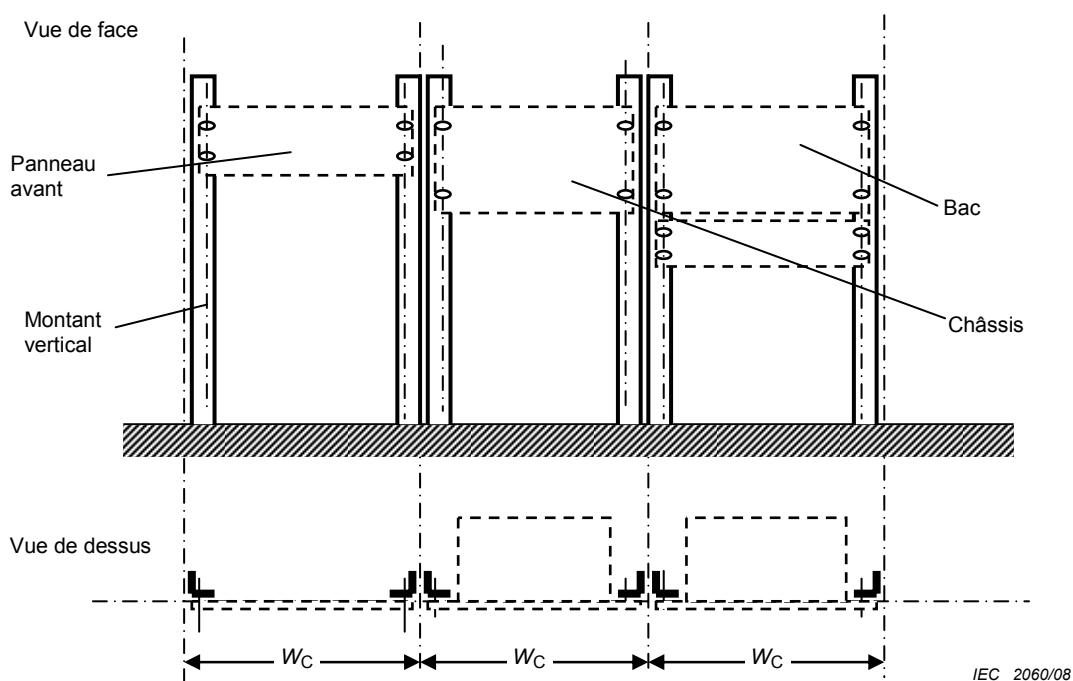
Figure 5 – Ensemble de bâtis
